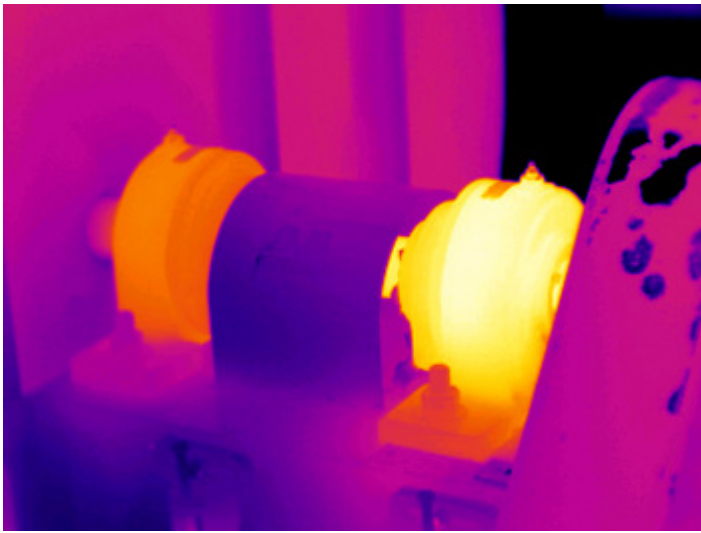
Túlmelegedett csapágyház
