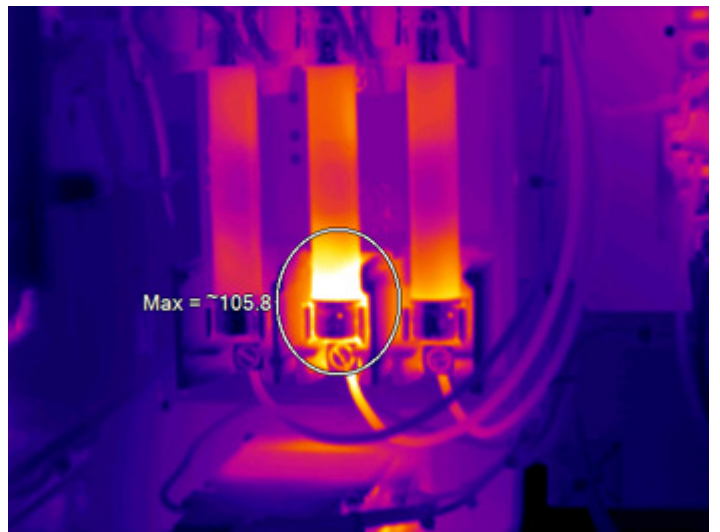
Biztosíték melegedése
